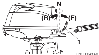
1. Levier inverseur
