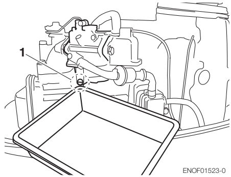
1. Vis de vidange du carburateur
